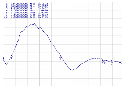
V.S.W.R
