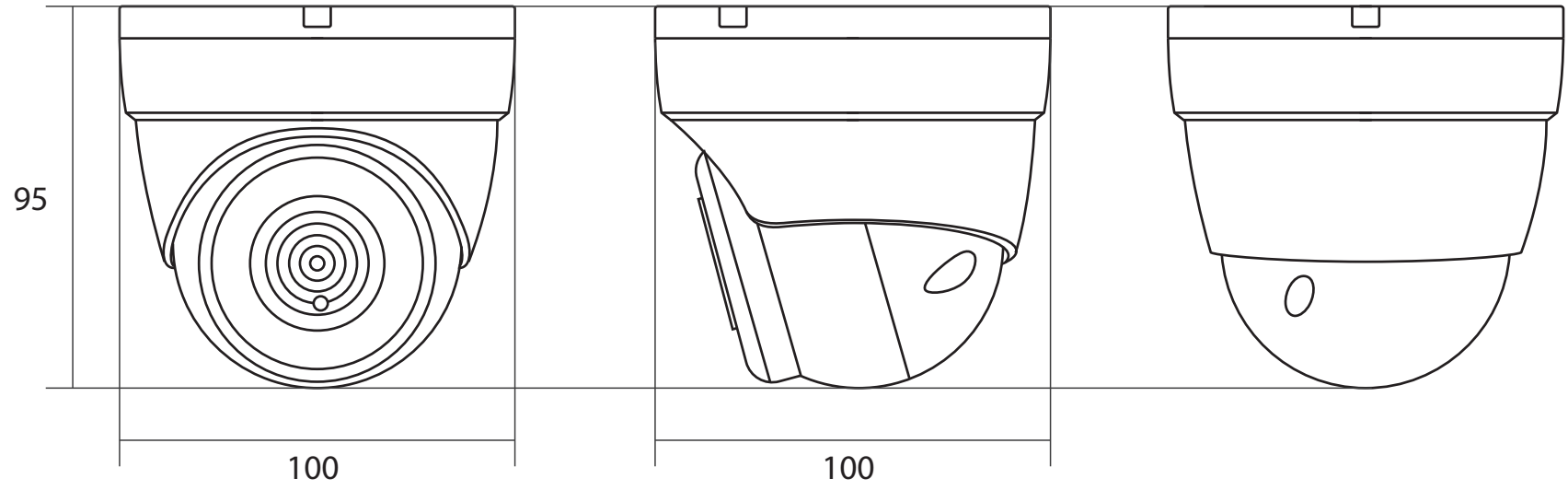
図名 500万画素 AHDシリーズ 図番 WTW-ADR48GAW WIRELESS TSUKAMOTO CO., LTD
