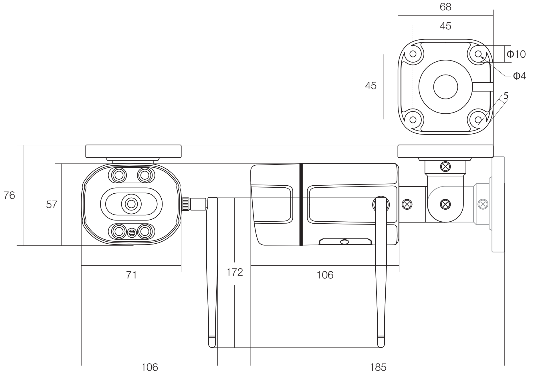
図名 500万画素 WiFi カメラ 図番 WTW-EGR2319GFBX WIRELESS TSUKAMOTO CO., LTD
