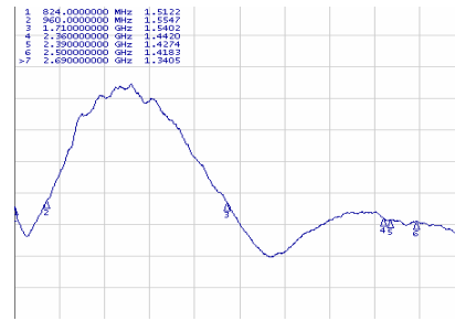
V.S.W.R
